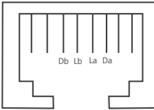
Anschlussbelegung am Analogport
